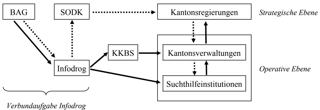
Abbildung 2: Bottom-up-Vorgehensweise
